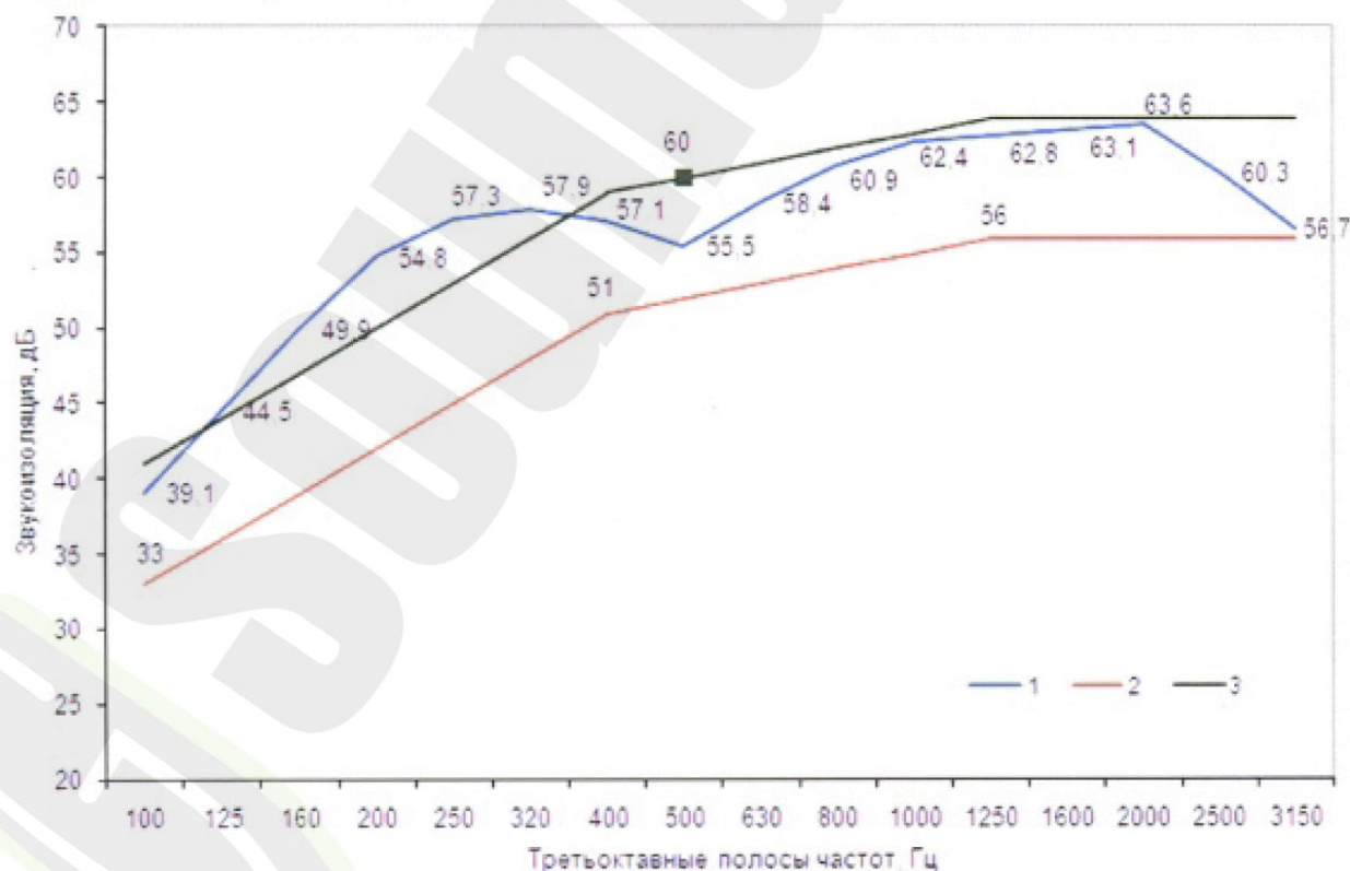
Рис.2. Определение индекса изоляции воздушного шума:
