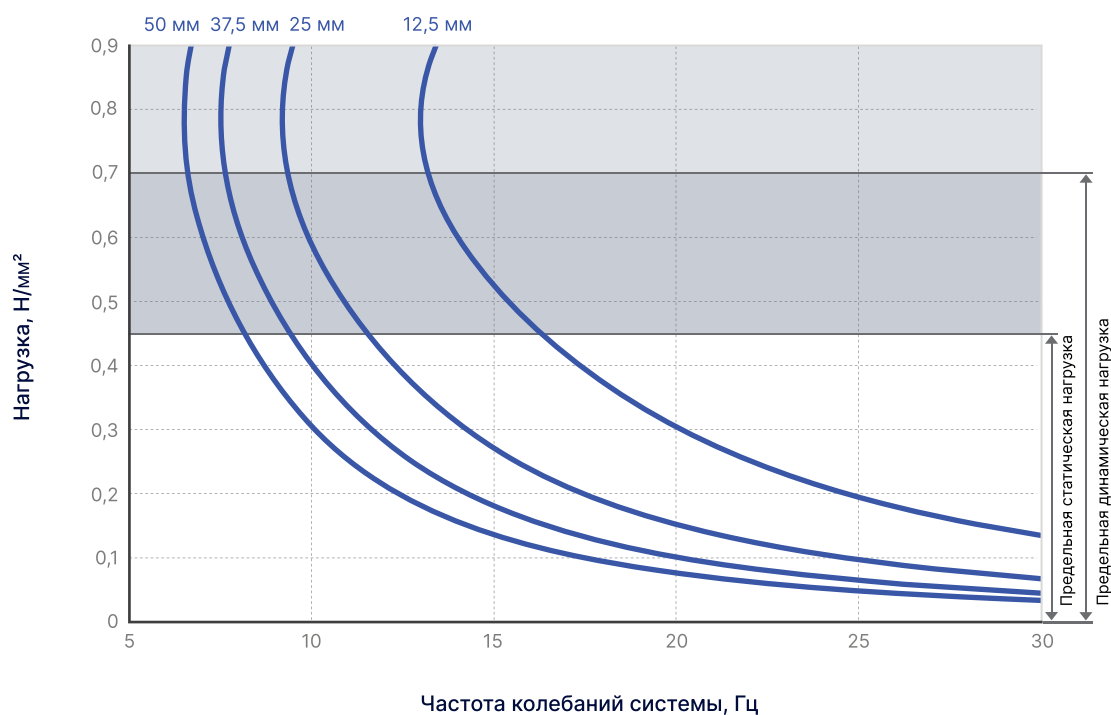
Диаграмма собственной частоты системы под нагрузкой
