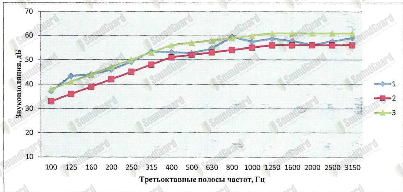
Рисунок 2. Частотные характеристики каркасной системы звукоизоляции перегородки « Оптима»;
