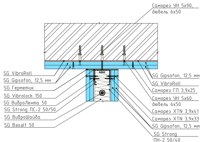
18 Узел сопряжения бескаркасной системы с каркасной системой звукоизоляции стены (внутренний угол)
