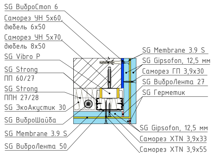
13 Узел сопряжения каркасной системы с бескаркасной системой звукоизоляции стены (наружный угол)
