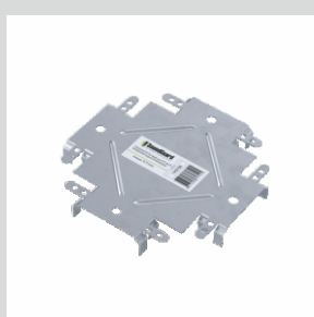
Соединитель профилей SoundGuard одноуровневый Каб для ПП 60/27
