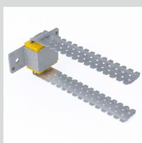
Виброизоляционное крепление SoundGuard Vibro PL (50 шт./уп)
