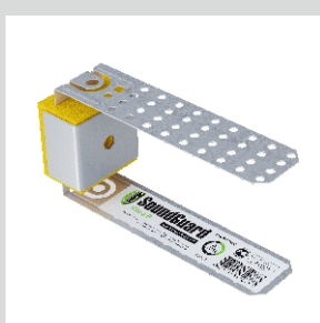
Виброизоляционное крепление SoundGuard Vibro P (60 шт./уп)
