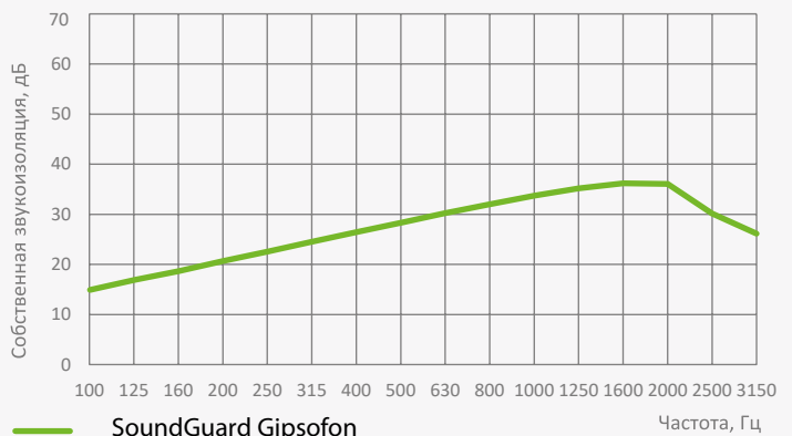
График собственной звукоизоляции воздушного шума Gipsofon (расчетно)
