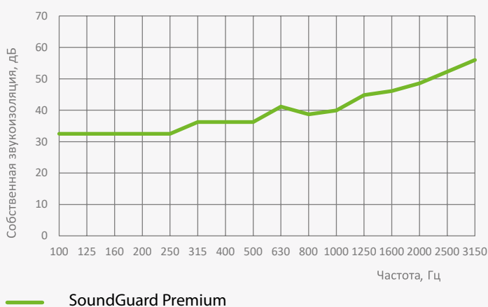
График собственной звукоизоляции воздушного шума SoundGuard Premium (измерено)
