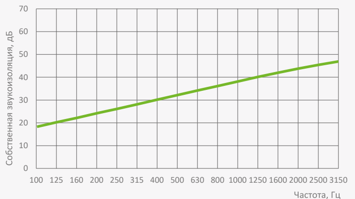
График собственной звукоизоляции воздушного шума SoundGuard ШумоЩит (расчетно)
