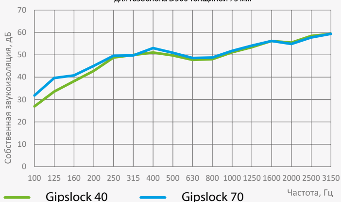
График собственной звукоизоляции воздушного шума SoundGuard Gipslock (расчетно *)
